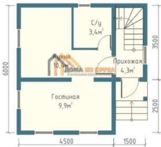
План 1-го этажа
